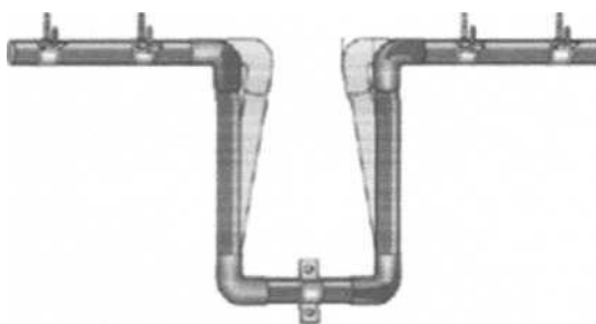
Рисунок 3 - П-образные компенсаторы
